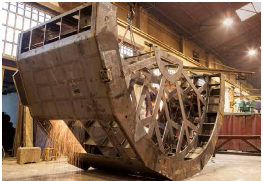
Teil eines Generatorgestells für ein Wasserkraftwerk mit einem Durchmesser von fünf Metern
